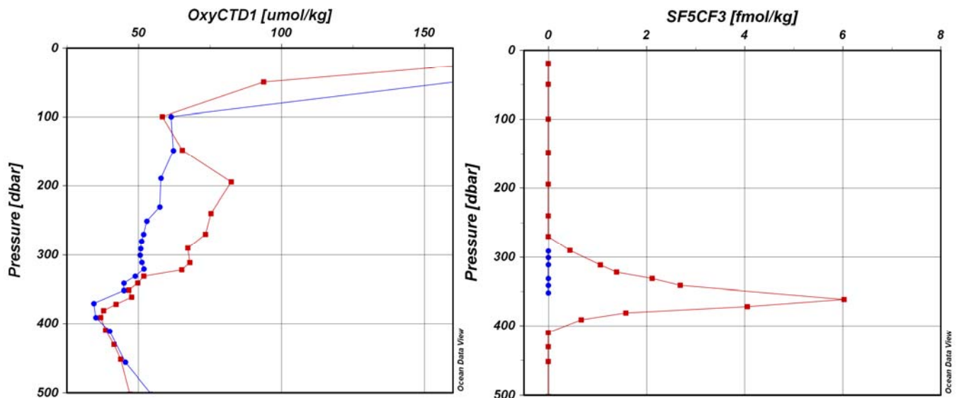
Abb.: Vertikalprofile der beiden Stationen 19 (Rot) und 20 (Blau). Links die Sauerstoffkonzentration (noch nicht abschließend kalibriert). Rechts die Konzentration des Tracers. Auf Station 20 war kein Tracer nachweisbar.
