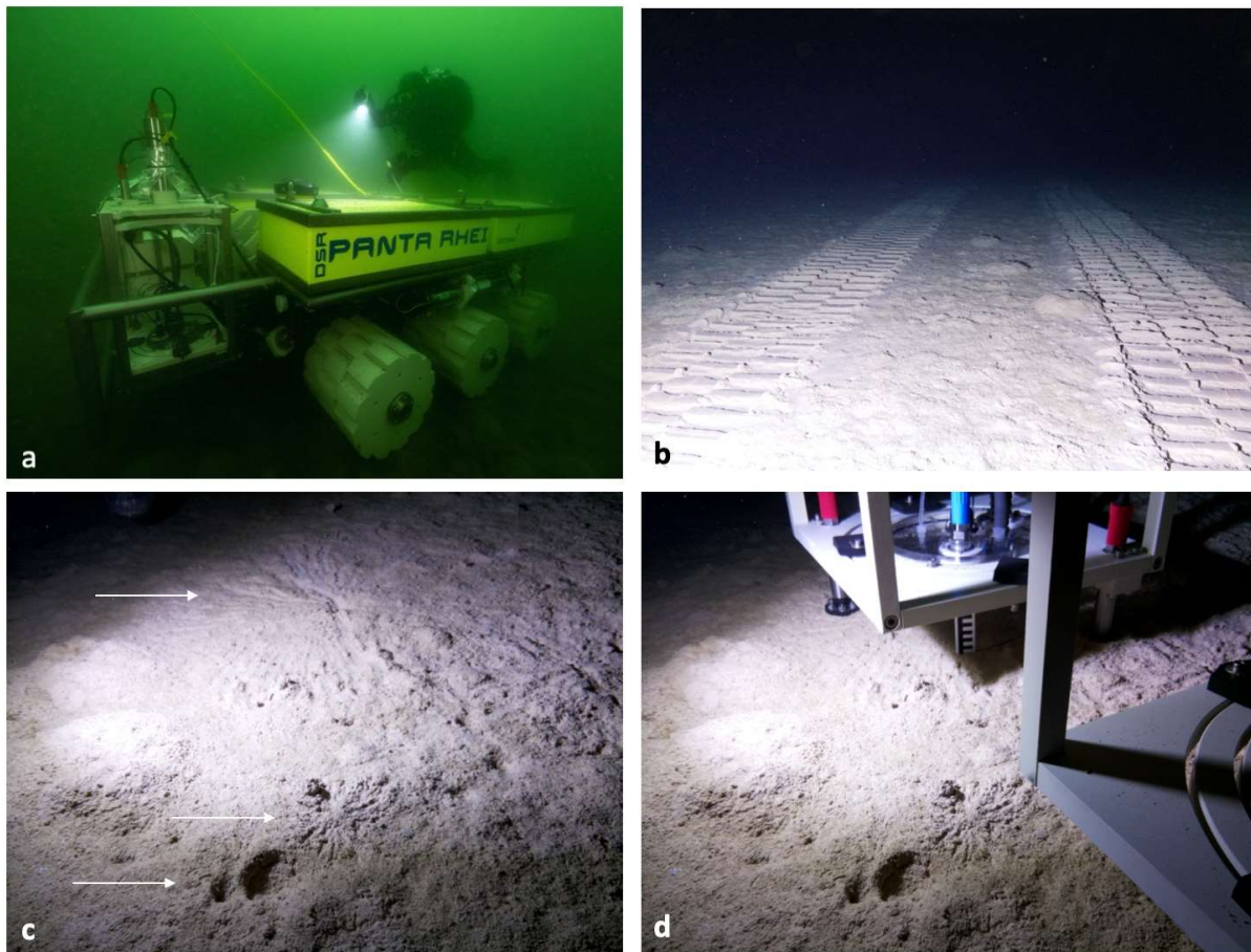
(a) Erste Tests des DSR Panta Rhei in der Ostsee. An der Vorderseite des Rovers befinden sich zwei Fluxkammern zur Bestimmung der TOU. (b) Der Rover wurde an der Station E1 vor den Kapverden in einer Wassertiefe von 3600 m ausgesetzt. Nach dem Absetzen des DSR Panta Rhei auf dem Meeresboden verließ er seinen Landeplatz. Das Foto zeigt den Blick nach hinten, wo die Radspuren zu sehen sind. (c) Unberührte Tiefseesedimente vor der Strömungsmessung. Spuren von Tieren (Pfeile) sind an der Sedimentoberfläche leicht zu erkennen. (d) Dieselbe Sedimentoberfläche wie in (c), aber mit eingesetzter Fluxkammer zur Bestimmung des TOU.
