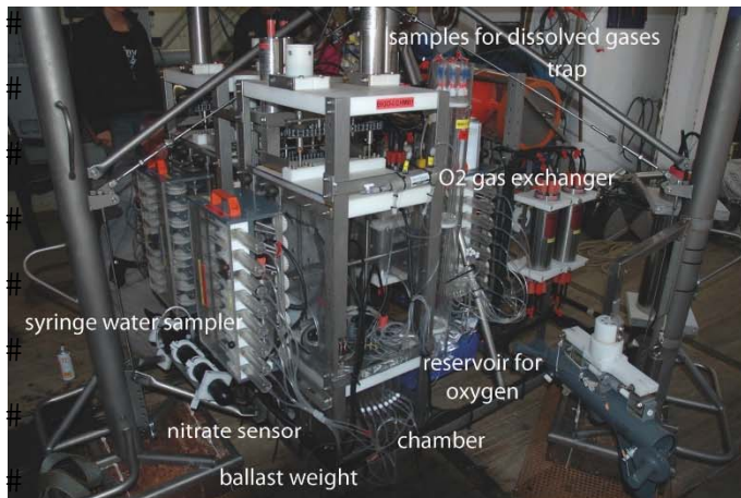
Abb.1: links, wissenschaftliche Nutzlast des BIGO Landers; rechts oben, Bergen des BIGO Landers - das Risiko, dass die weichen Sedimente dabei aus den Kammern auslaufen ist hoch; rechts unten, Ausschnitt der Sediment-Oberfläche in einer der beiden Kammern. Die weißlichen Filamente stellen Schwefelbakterien dar. (Photos: S. Sommer & I. Mekelnburg)
