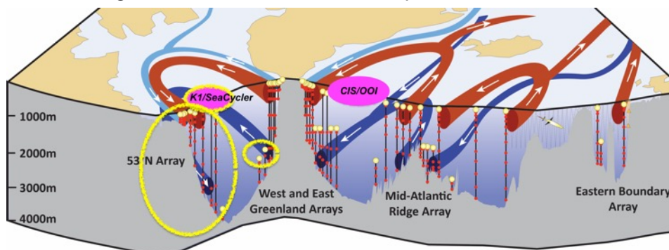
Schematik der OSNAP Messinstallation die hauptsächlich aus Verankerungen in ausgewählten Regionen besteht. (Schematik: OSNAP)
