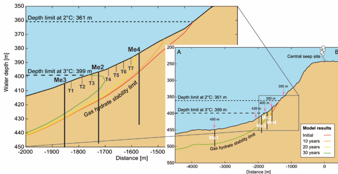
Abb. 8: West-Ost Profil am oberen Kontinentalrand im Bereich der oberen Gashydratstabilitätsgrenze, bei 2° und 3° C des Bodenwassers und Bohrlokalationen.
