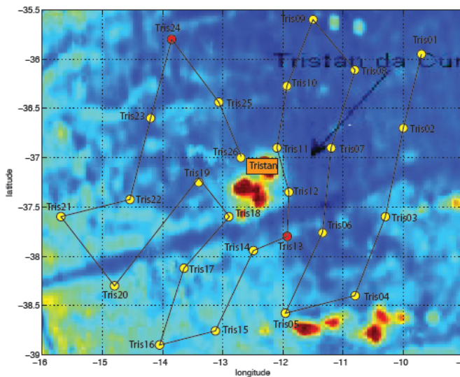
Abbildung 1: Links: Der Stationsplan um Tristan da Cunha. Gelb markiert sind Stationen die sowohl mit OBS und OBMT belegt sind, rot Stationen an denen nur ein OBMT ausgelegt werden. Rechts: Aussetzen der ersten OBM Station in der Nacht von Sonntag, den 22.1. auf Montag den 23.1.
